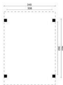
Plattegrond enkele carport
