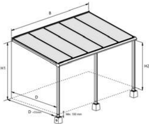
Tekening 3D
