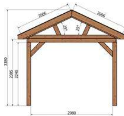
Zijaanzicht L
