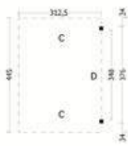
Uitbreidingsset XL
