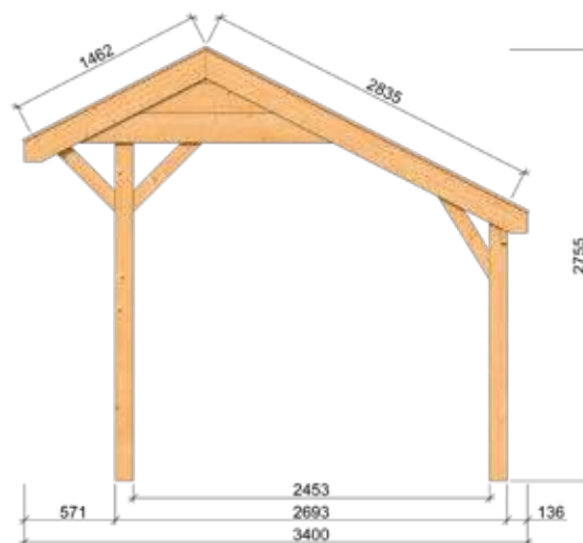
vue latérale
