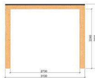
vue latérale
